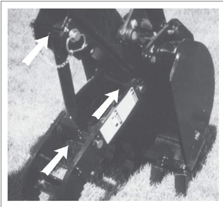
Fig. 8 PIVOT PINS
